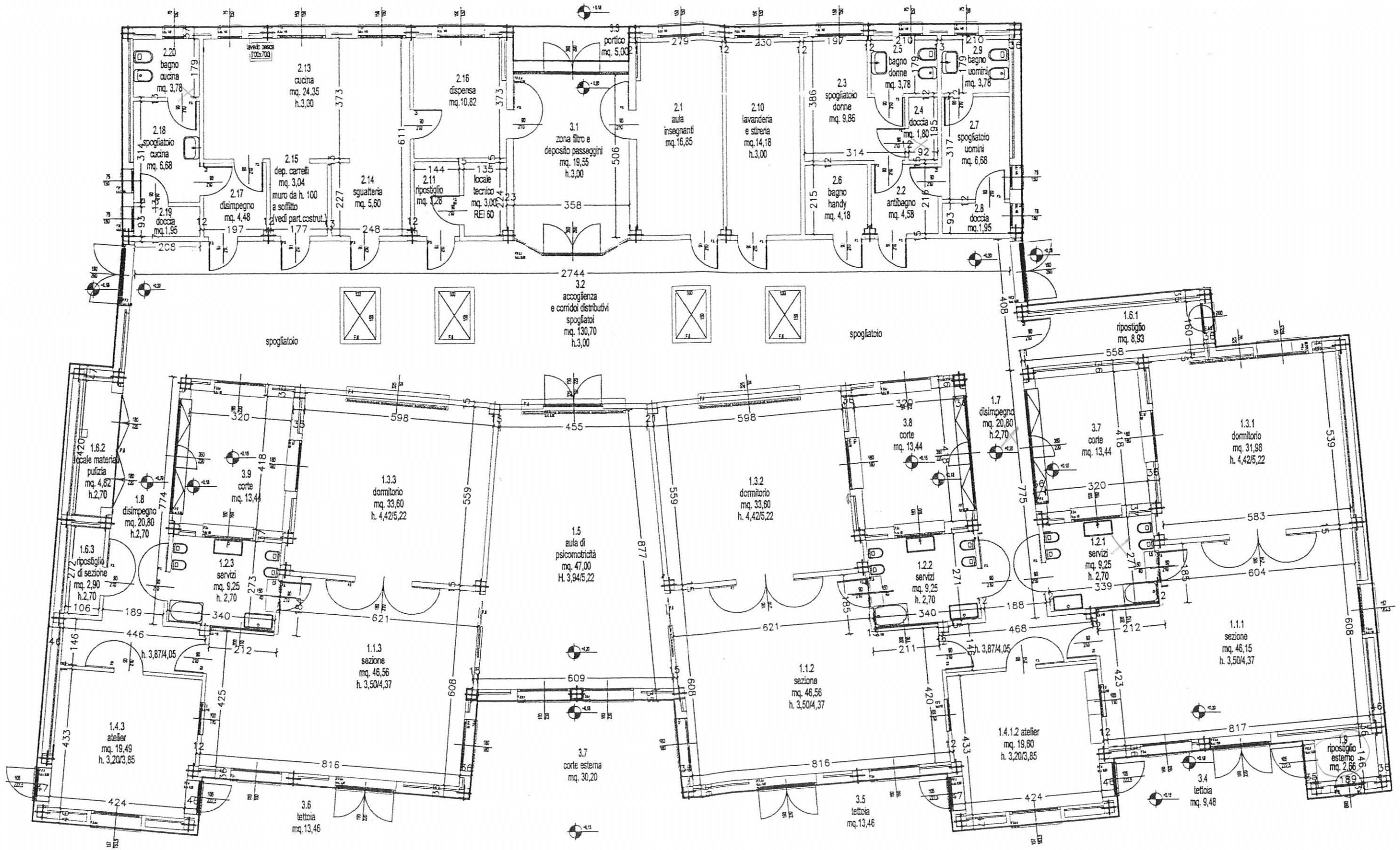
ASILO NIDO - ARGELATO PIANTA PIANO TERRA NON IN SCALA
