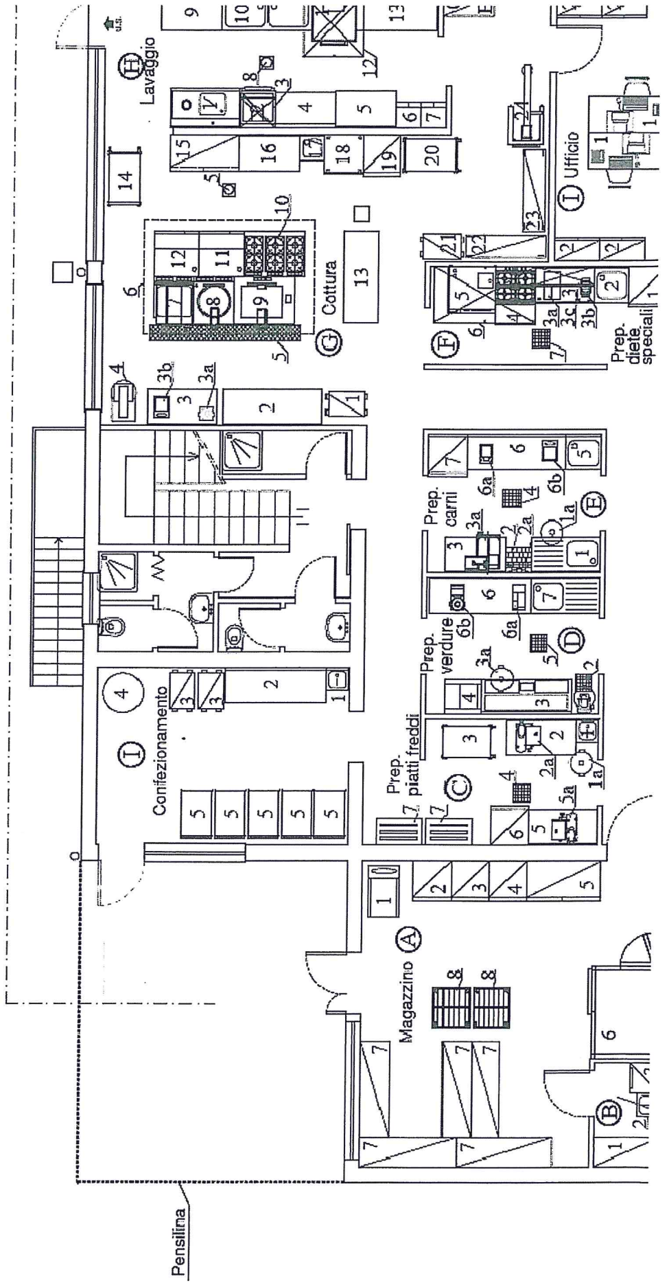
PIANTA PIANO TERRA (SCALA 1:50)
